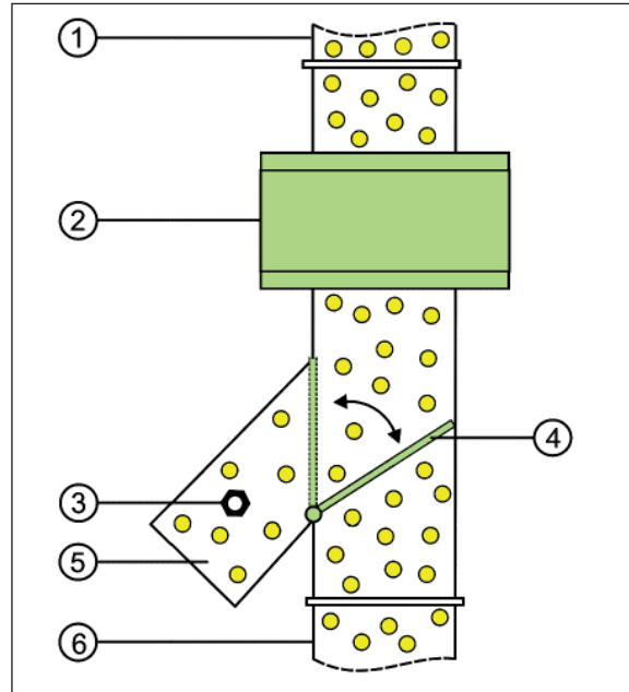
1)Đầu vào 2)Cuộn dò 3) Tụ chất kim loại 4)Bẫy sập 5)Đầu ra tụ chất 6)Đầu ra nguyên liệu
